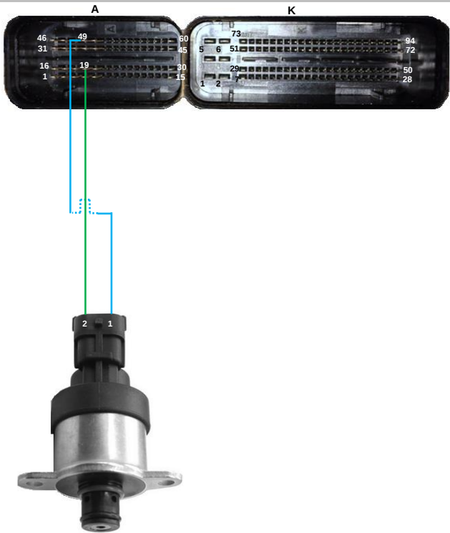
Válvula dosadora de combustível Mprop
