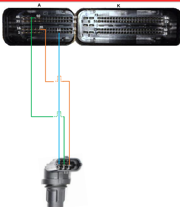
Sensor de fase
