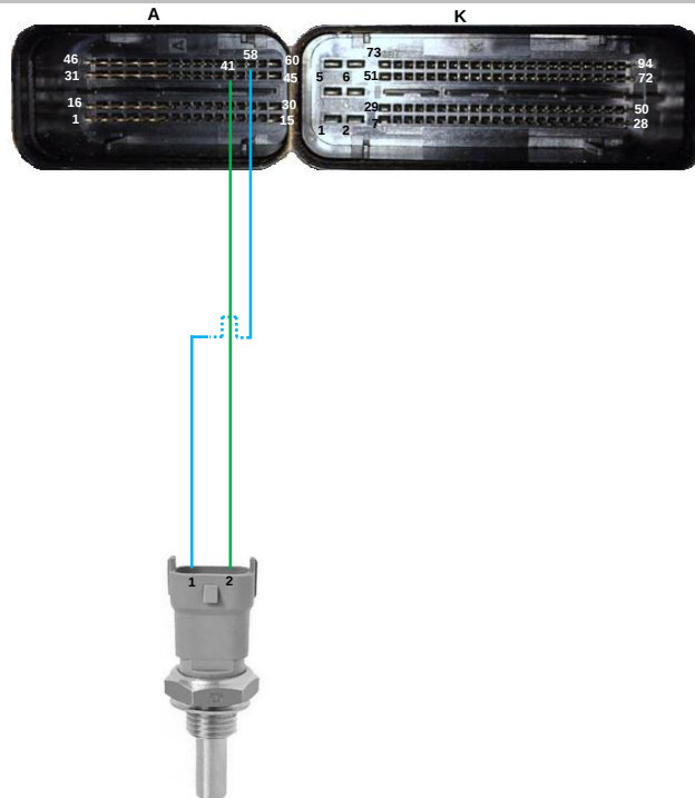
Sensor de temperatura do motor
